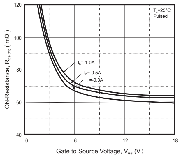
Fig.4 - R_{DS(ON)} - V_{GS}
